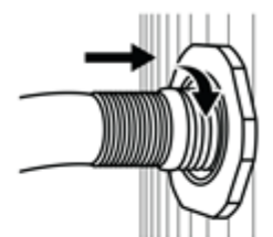
4. Système de drainage en position ouverte (tourner le tuyau et le raccord sur ¼ de tour en sens horaire et enfoncez le à mi-chemin pour ouvrir le robinet).
